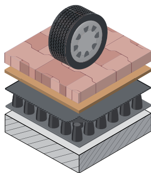
Opbouw Nophadrain Parkeerdaksysteem
