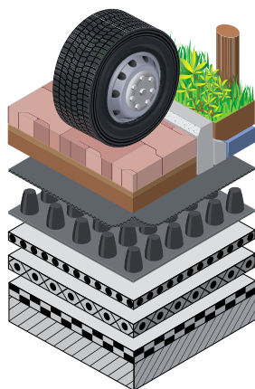
Opbouw Nophadrain Parkeerdaksysteem - vrachtverkeer
