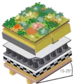
Opbouw Nophadrain Extensief Groendaksysteem - Hellenddak
