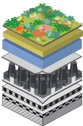
Aufbau Nophadrain Extensiv Grunddachsystem mit ND 6+1v
