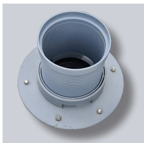
ND AFC-100 Instelbare Stuwingsregelaar
